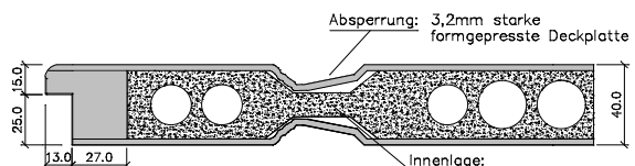
Überschlag rund (WR-Tür)
