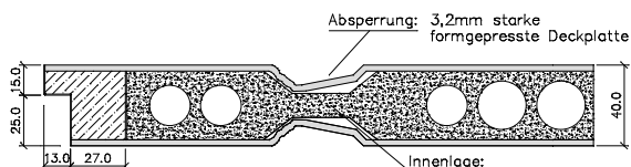
Überschlag eckig (WF-Tür)
